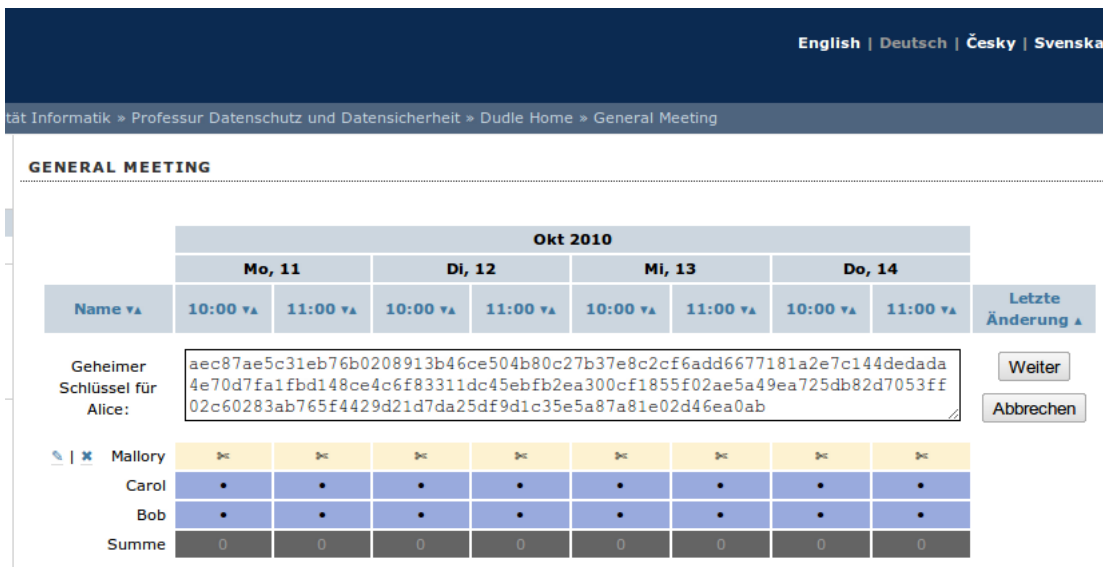
Abbildung 5.17.: Interface, welches zur Schlüsseleingabe während der Abstimmungsphase auffordert
