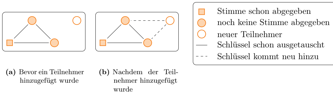
Abbildung 4.11.: Schlüsselgraph vor und nach dem dynamischen Hinzufügen von Teilnehmern
