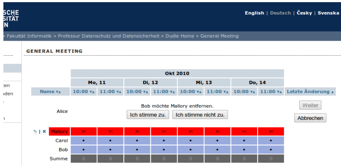
Abbildung 5.18.: Interface, welches über das dynamische Entfernen eines Teilnehmers informiert. Bob möchte Mallory aus der Umfrage entfernen und hat deshalb die mit Mallory gemeinsamen symmetrischen Schlüssel zum Umfrageserver geschickt. Da Alice erst später abstimmt, wird sie bei der Stimmenabgabe gefragt, ob sie dieser Entfernung zustimmt und auch ihre mit Mallory gemeinsamen Schlüssel offenlegt. Die Umfrage kann nur abgeschlossen werden, wenn alle Teilnehmer dem Entfernen zustimmen oder Mallory selbst mit abstimmt.
