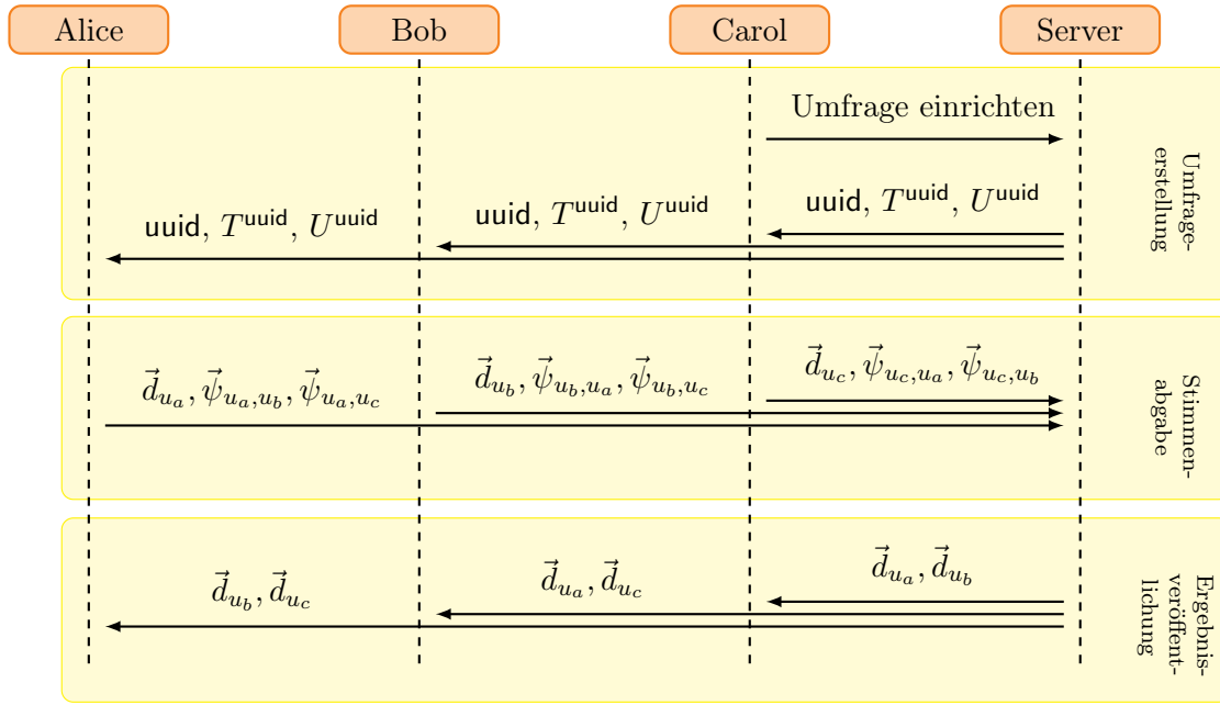
Abbildung 4.10.: Kommunikationsschritte des Protokolls, wenn ein Schlüsselvereinbarungsprotokoll verwendet wird
