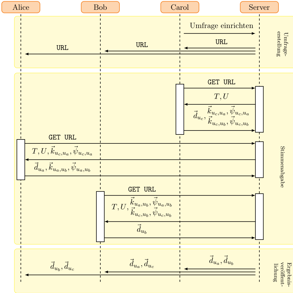
Abbildung 4.9.: Kommunikationsschritte des Protokolls, wenn ein Schlüsseltransportprotokoll verwendet wird. Die Darstellung beinhaltet nur, welche Daten zwischen den Entitäten ausgetauscht werden. Insbesondere wurde auf die Darstellung der Verschlüsselung und der Signatur aus Lesbarkeitsgründen verzichtet. Die verschlüsselten Verfügbarkeitsvektoren ( \vec{d}_u ) sind jeweils von ihren Sendern digital signiert. Die Schlüsselvektoren der Paarbeziehungen ( \vec{k}_{u,u'} ) sind für den jeweils anderen Partner asymmetrisch verschlüsselt. Die verschlüsselten Schlüsselvektoren, sowie die Commitments ( \vec{\psi}_{u,u'} ) sind von ihren Sendern digital signiert. Ein Beispiel für eine solche Nachricht ist in Gleichung (4.30) auf der vorherigen Seite dargestellt. Die URL ist die URL, unter welcher die Umfrage aufgerufen werden kann.
