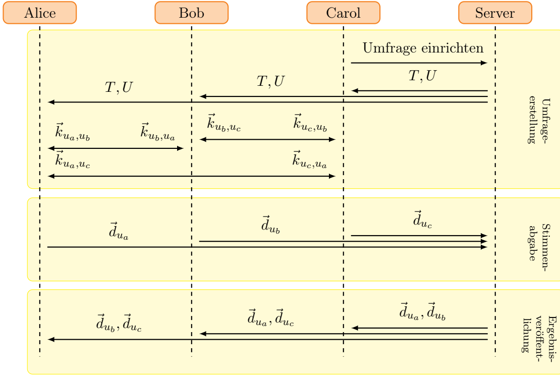
Abbildung 4.2.: Phasen des Protokolls
