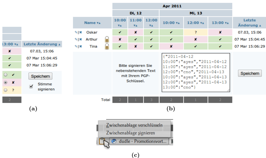
Abbildung 5.13.: Interface, um dem Verfügbarkeitsvektor eine digitale Signatur anzuhängen
