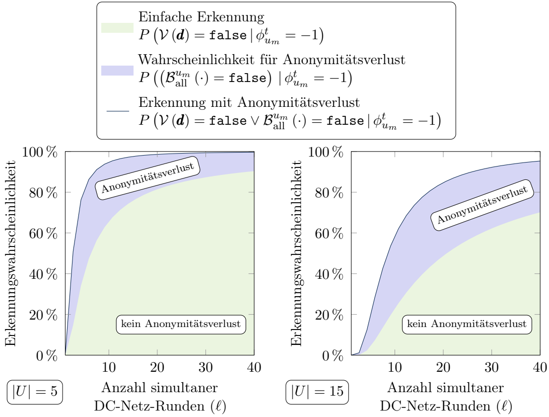
Abbildung 4.7.: Untere Schranken für die Wahrscheinlichkeit, einen (-1) -Angriff zu erkennen
