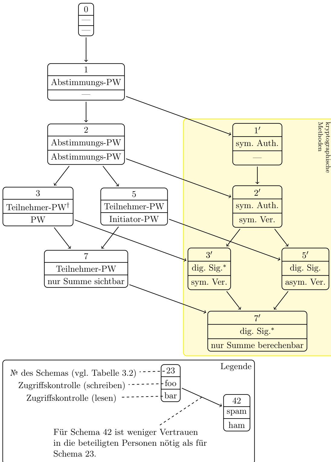
Abbildung 3.1.: Diagramm über das notwendige Vertrauen, welches den verschiedenen Entitäten entgegengebracht werden muss.
