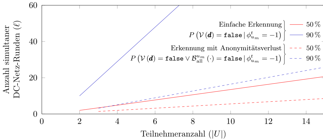
Abbildung 4.8.: Abhängigkeit zwischen der Anzahl der Teilnehmer und der Anzahl der DC-Netz-Runden bei fester Erkennungswahrscheinlichkeit
