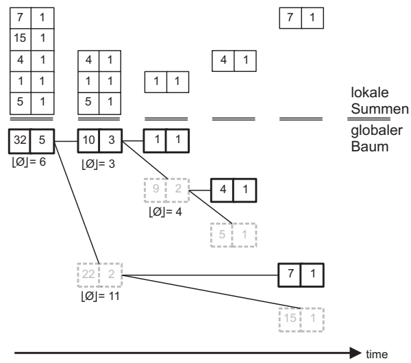
Abbildung 6: Abarbeitungsbaum bei der Kollisionsauflösung
